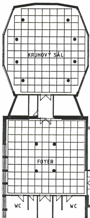
DK METROPOL PÚDORYS 1.NP - VÝŘEZ 1:200
